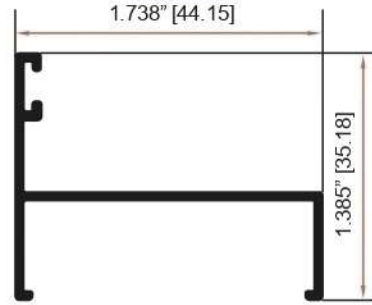
BATIENTE LATERAL SIN VENA 5056
