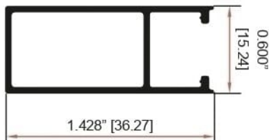
CERCO CHAPA VENTANA 2" 2086
