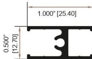
INTERMEDIO PARA CUADRICULA 1" 12021
