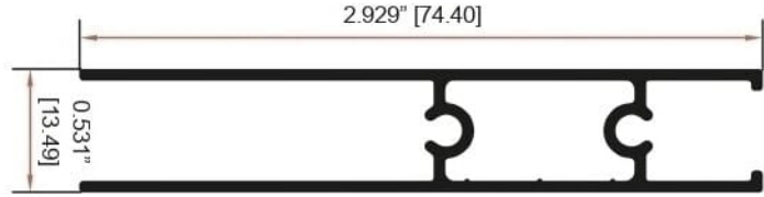
ZOCLO PUERTA DE 2" 12105
